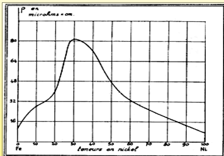
Variazione della resistività: curva in funzione del contenuto di nichel nelle leghe ferro-nichel (La Nature, 1934, Nickel alloys and their applications, P215)
